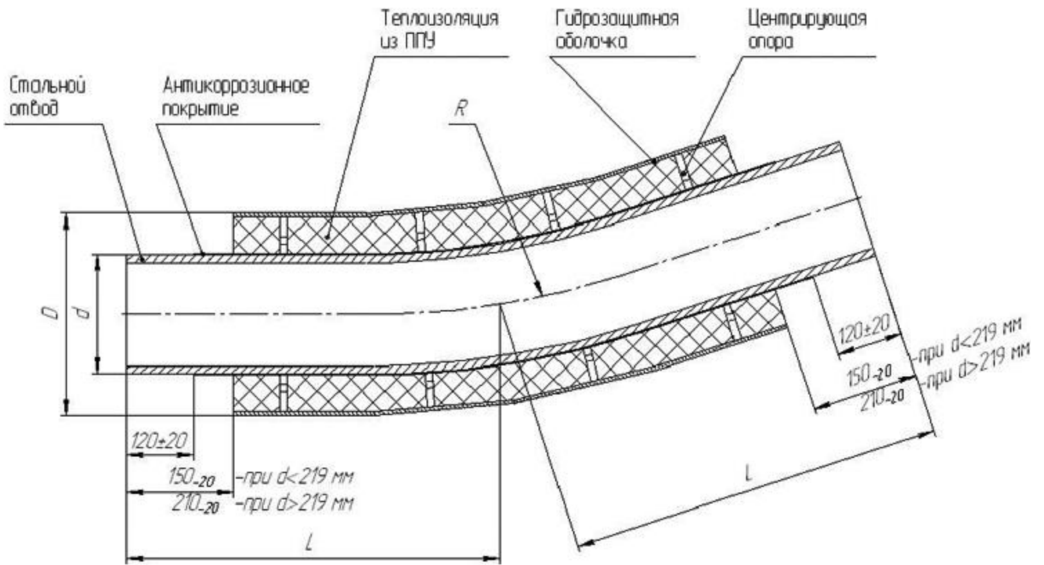
Рисунок А.2 - Конструкция тепловой изоляции отводов трубопроводов
