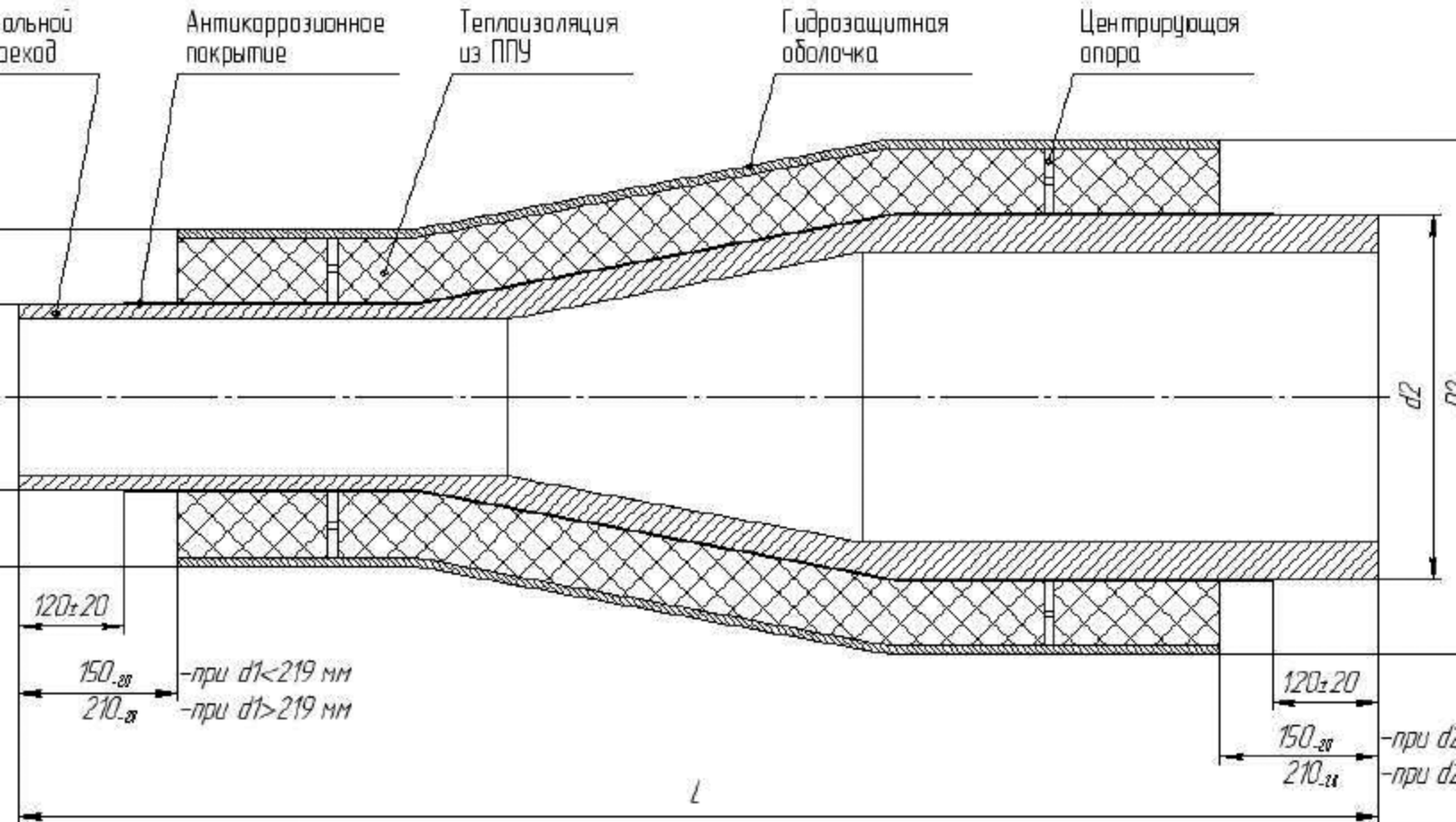
Рисунок А.3 - Конструкция тепловой изоляции переходов трубопроводов
