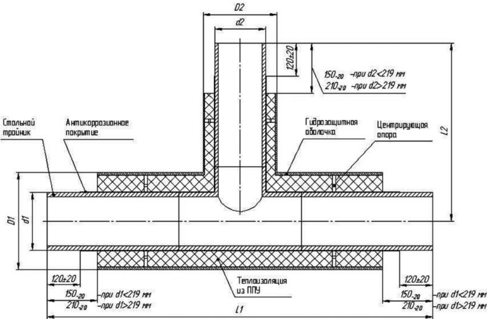
Рисунок А.4 - Конструкция тепловой изоляции тройников трубопроводов
